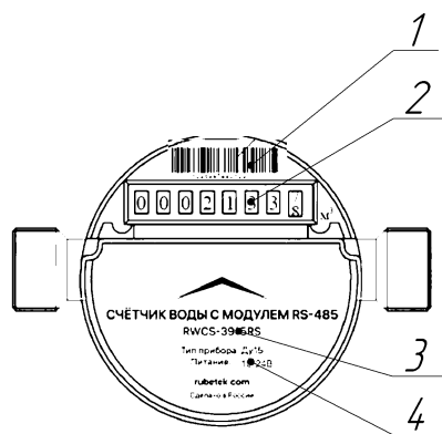
Рисунок 1 – Внешний вид счетчика с модулем (вид сверху)
