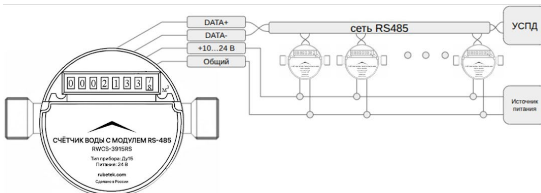
Рисунок 5 – Схема подключения модуля к линии RS-485
