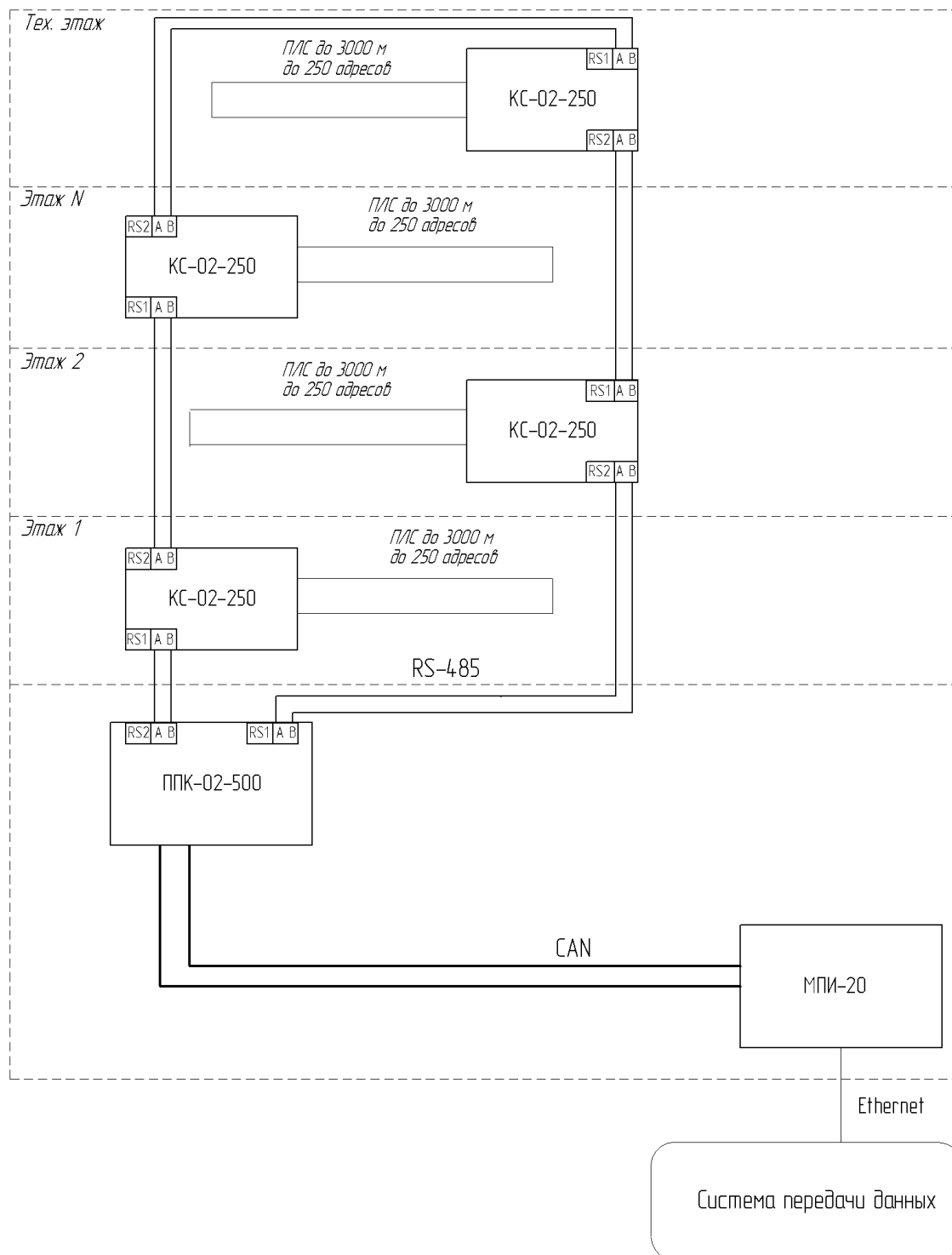
Рисунок 7 – Схема подключения контроллеров к ППК
