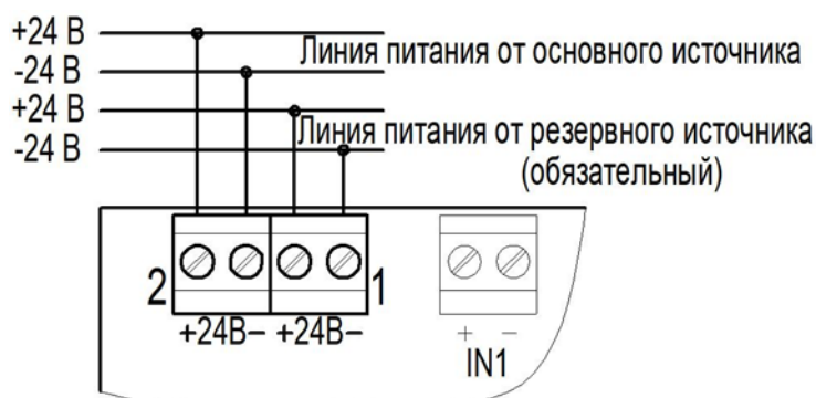
Рисунок 9 – Подключение питания
