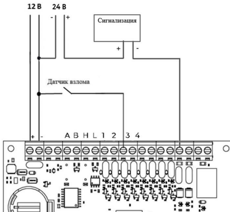
Рисунок 6 – Схема подключения датчика взлома для сигнализации с напряжением 24 В
