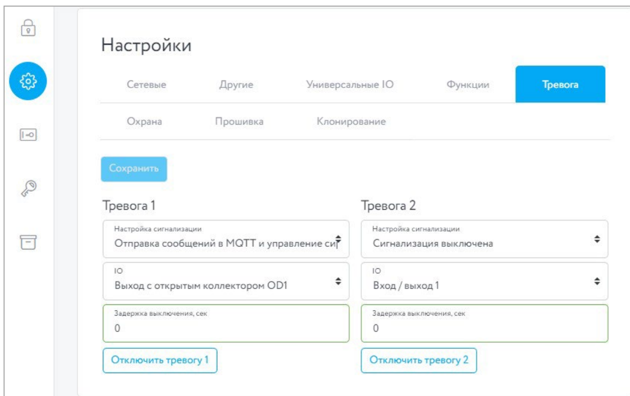
Рисунок 7 – Настройки вкладки «Тревога»
