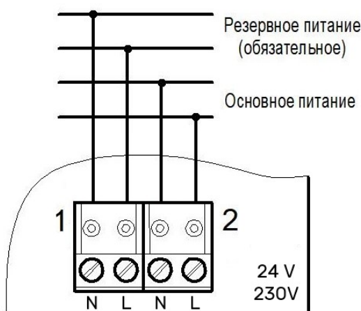
Рисунок 7 – Подключение питания
