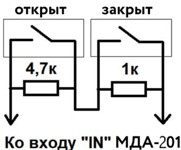
Рисунок 8 – Подключение внешних кнопок к клеммам входов
