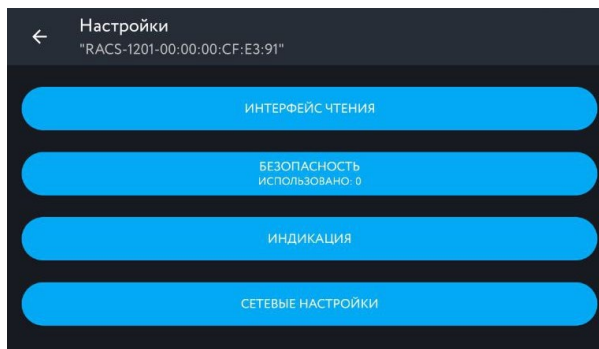
Рисунок 9 – Вкладка «Настройки»
