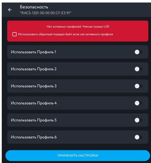
Рисунок 11 – Вкладка «Безопасность»
