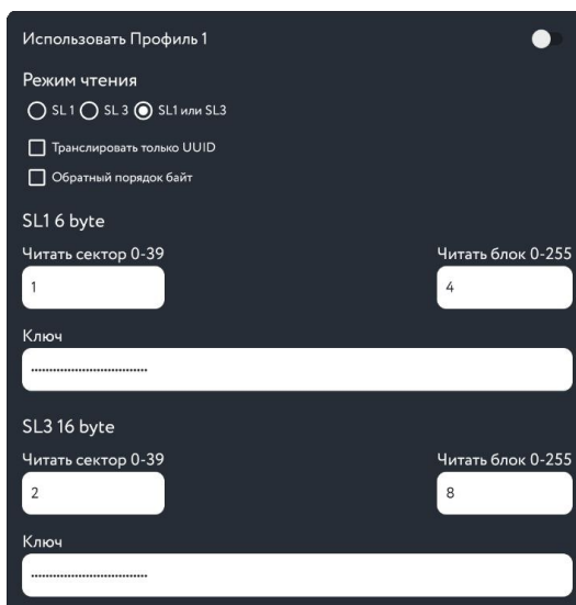
Рисунок 12 – Настройка профиля
