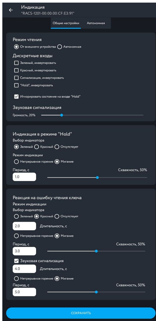
Рисунок 13 – Общие настройки
