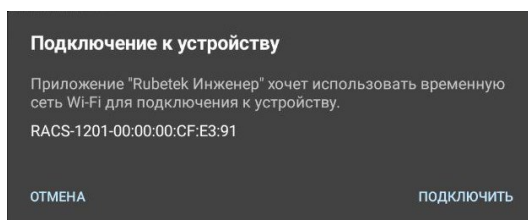
Рисунок 5 – Окно подтверждения
