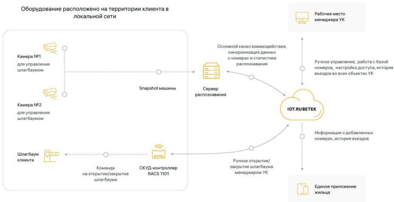
Рисунок 1 – Система распознавания автомобильных номеров Rubetek CarID
