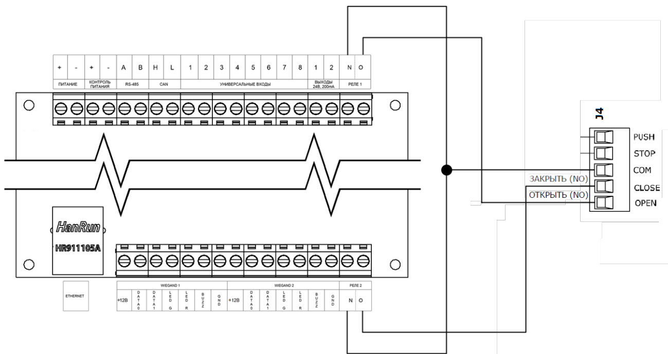
Рисунок 3 – Схема подключения шлагбаума к контроллеру системы
