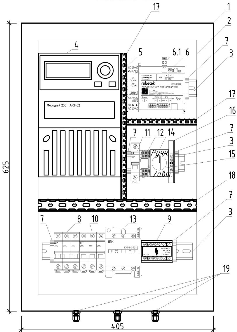
Рисунок 1.1 – Схема расположения составных частей
