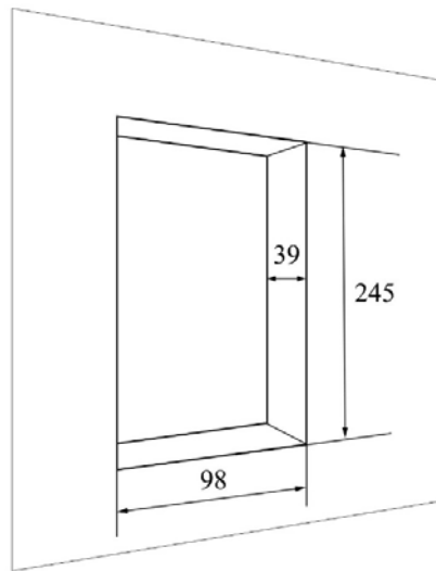
Рисунок 2 – Отверстие для врезного монтажа
