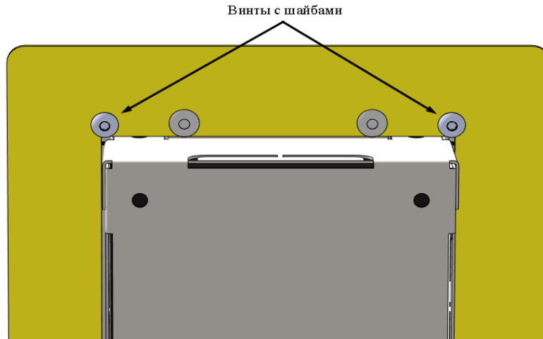
Рисунок 8 – Фиксация винтами к лицевой панели
