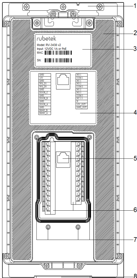
Рисунок 2 – Внешний вид панели (вид сзади)
