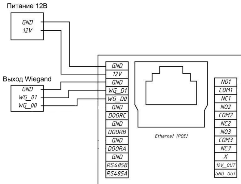
Рисунок 6 – Схема подключения считывателей
