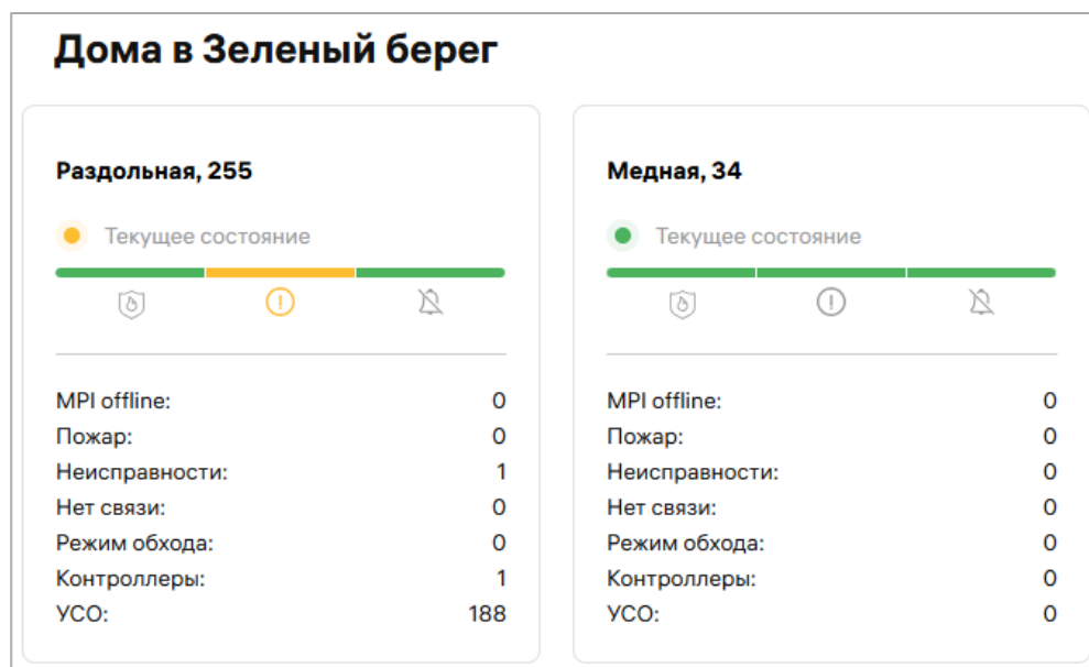
Рисунок 12 – Вкладка «Дома»
