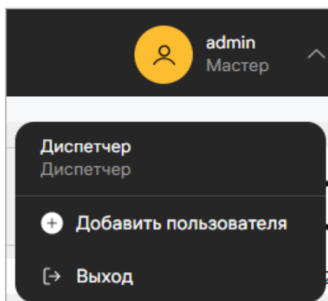
Рисунок 3 – Меню «Настройки»
