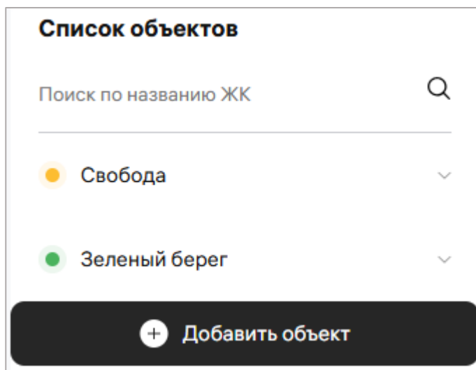
Рисунок 7 – Список объектов
