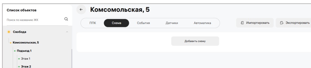
Рисунок 21 – Блок «Схема»
