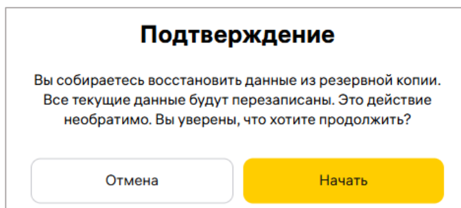
Рисунок 82 – Подтверждение восстановления
