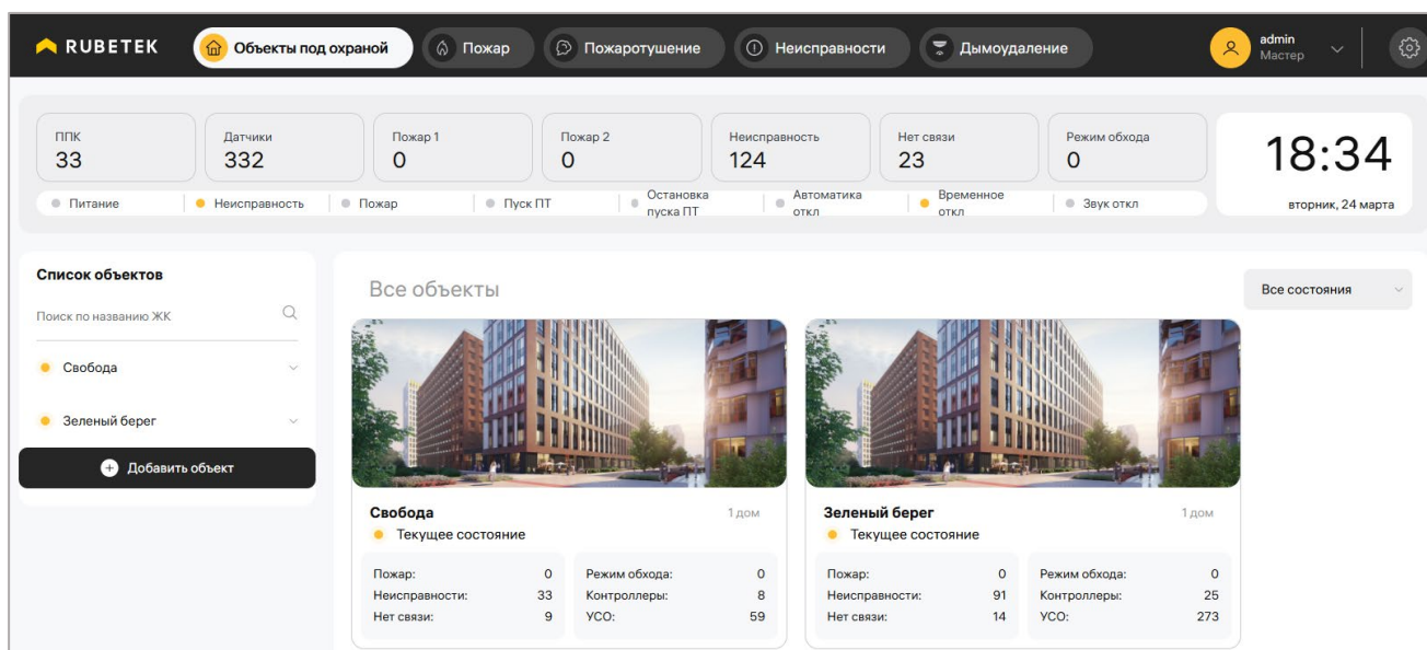
Рисунок 6 – Окно программы
