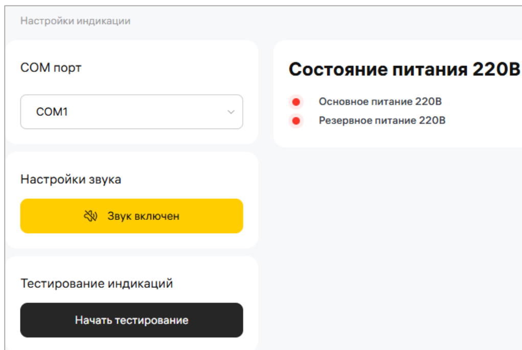
Рисунок 79 – Настройки индикации
