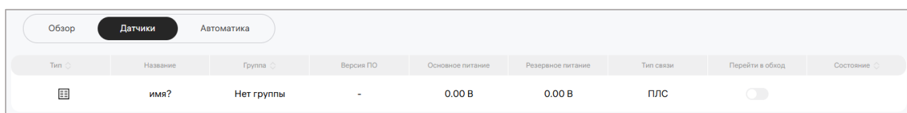
Рисунок 19 – Вкладка «Датчики»
