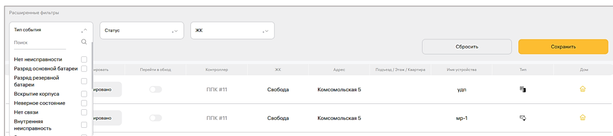
Рисунок 62 – Фильтрация неисправностей
