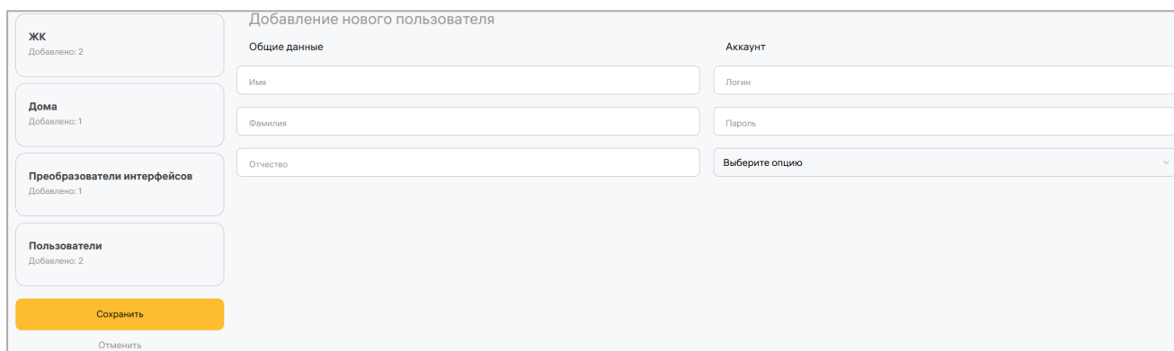
Рисунок 73 – Добавление пользователя
