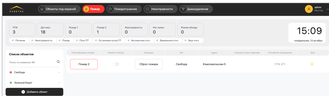
Рисунок 56 – Раздел «Пожар»
