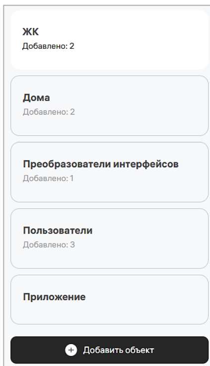
Рисунок 65 – Добавление объекта
