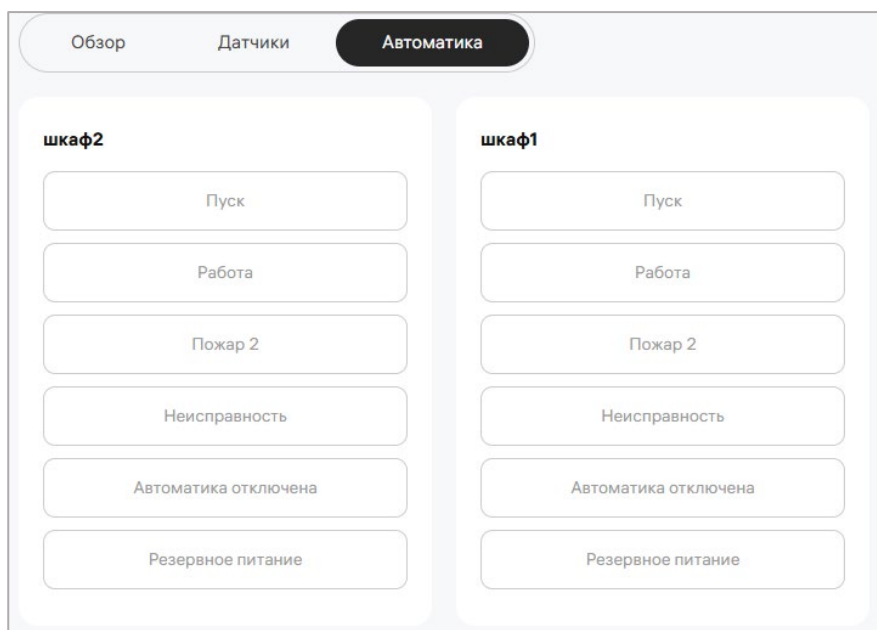
Рисунок 20 – Вкладка «Автоматика»
