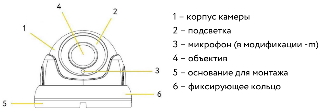
Рис. 1 – Внешний вид видеокамеры
