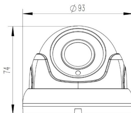
Рис. 2 – Габаритные размеры видеокамеры
