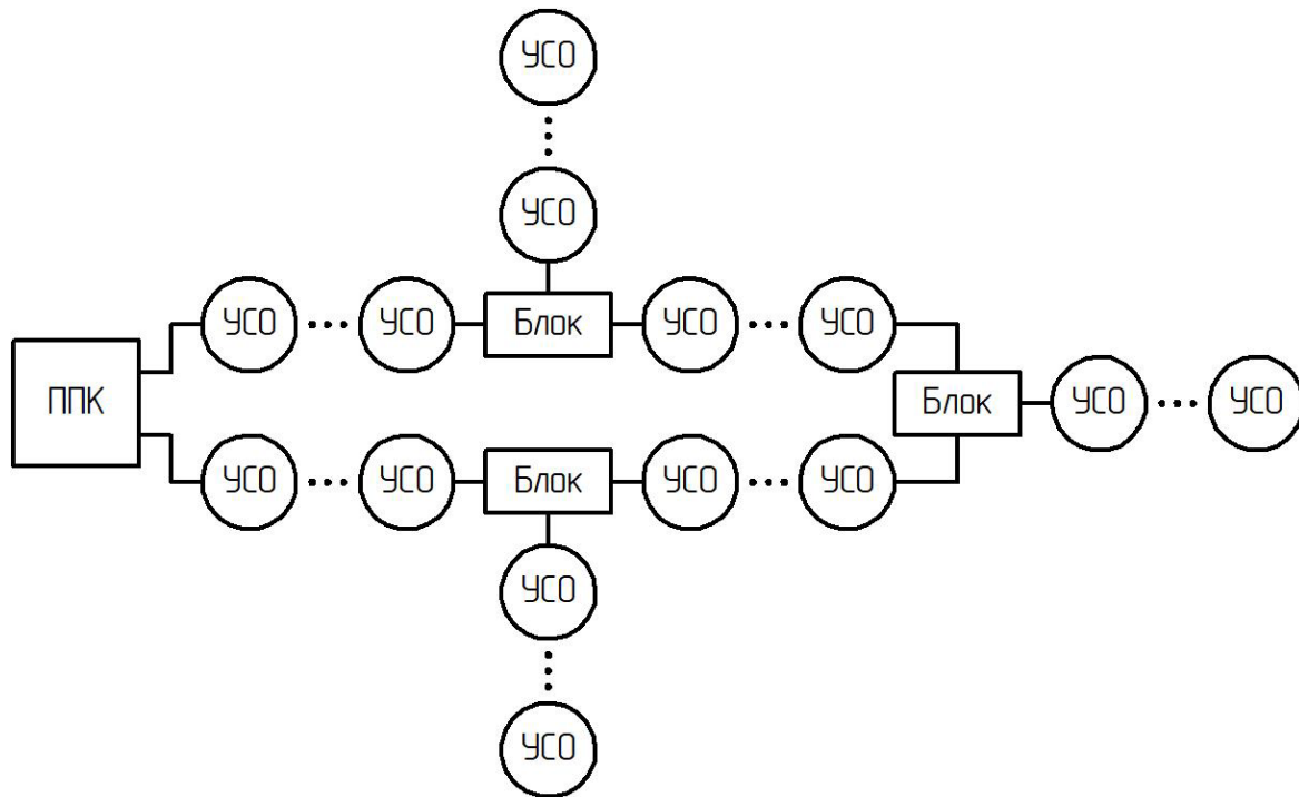
Рисунок 6 - Топология «Смешанная»
