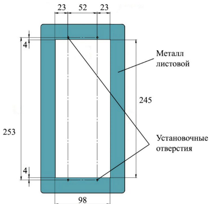
Рисунок 3 – Разметка установочных отверстий под заклепки
