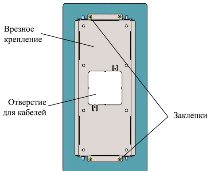
Рисунок 4 – Установка крепления в листовой металл
