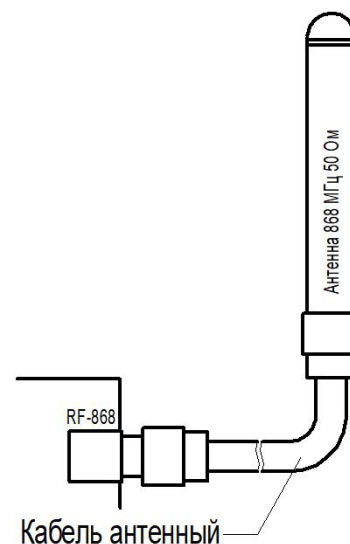
Рисунок 8 – Подключение антенны
