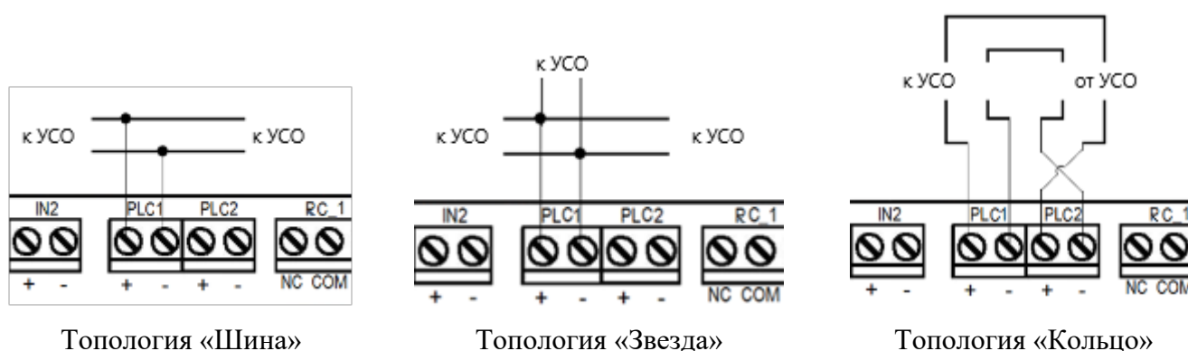
Рисунок 5 – Схемы подключения ПЛС
