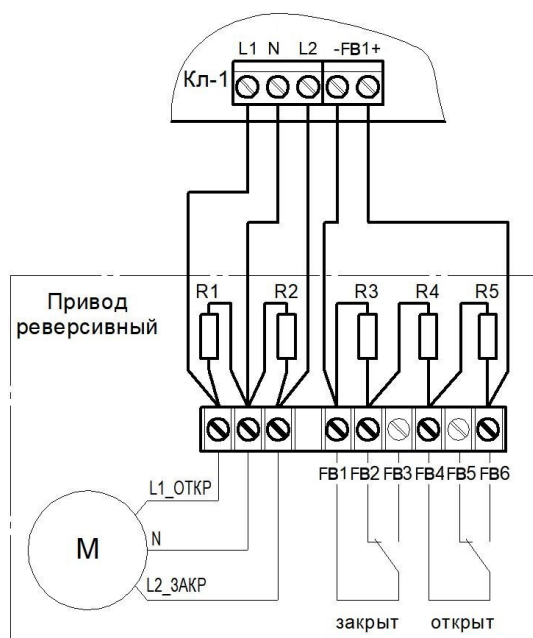
Рисунок 14 – Схема подключения реверсивного привода
