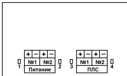
Рисунок 13 – Назначение клемм
