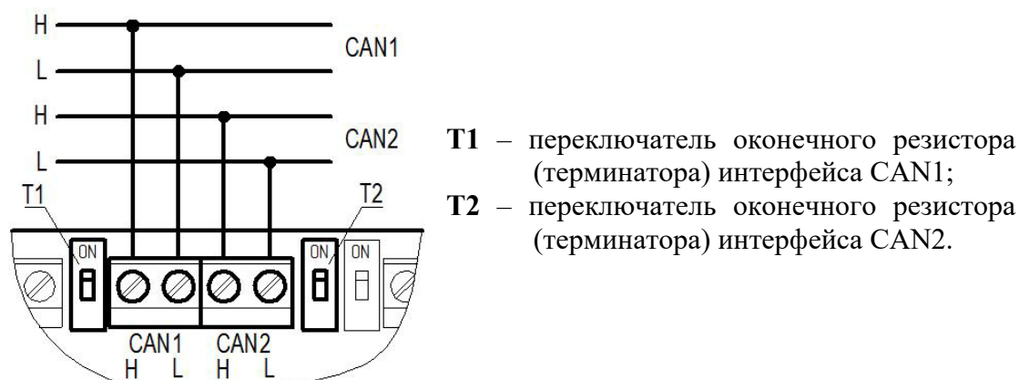
Рисунок 6 – Подключение CAN
