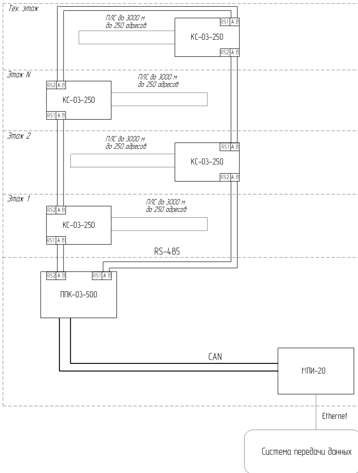
Рисунок 7 – Схема подключения контроллеров к ППК
