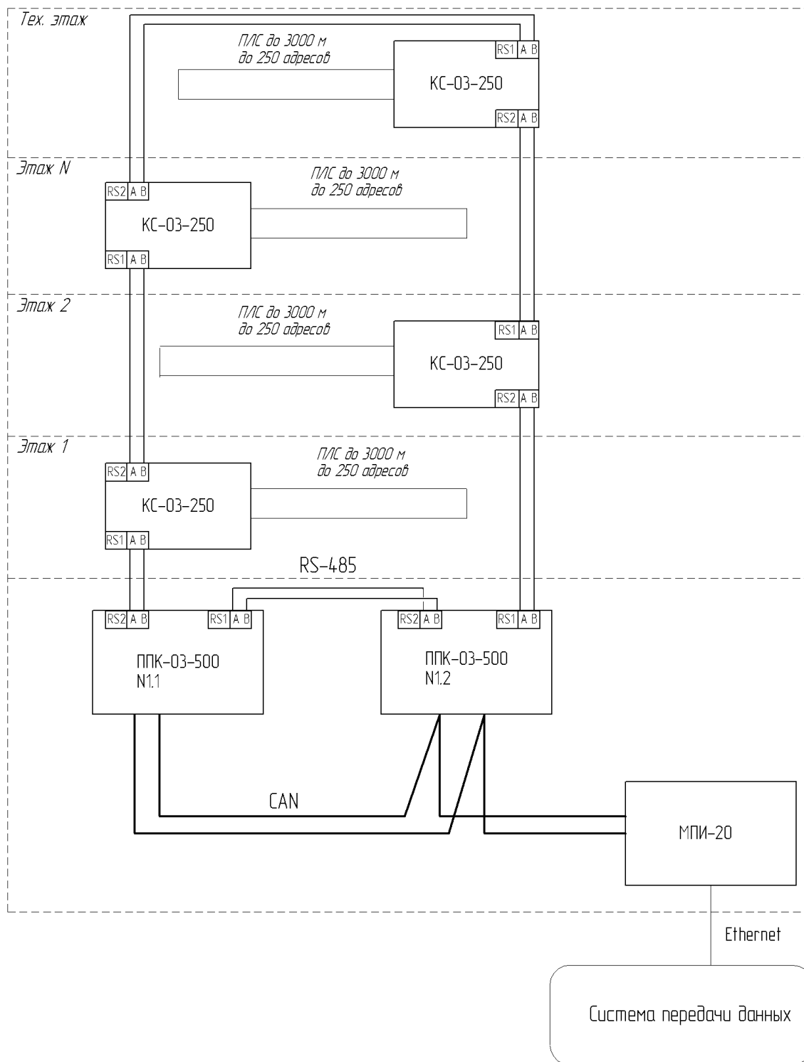
Рисунок 8 – Архитектура подключения двух ППК к шине RS-485
