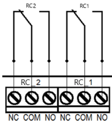
Рисунок 14 – Схема подключения к СК прибора
