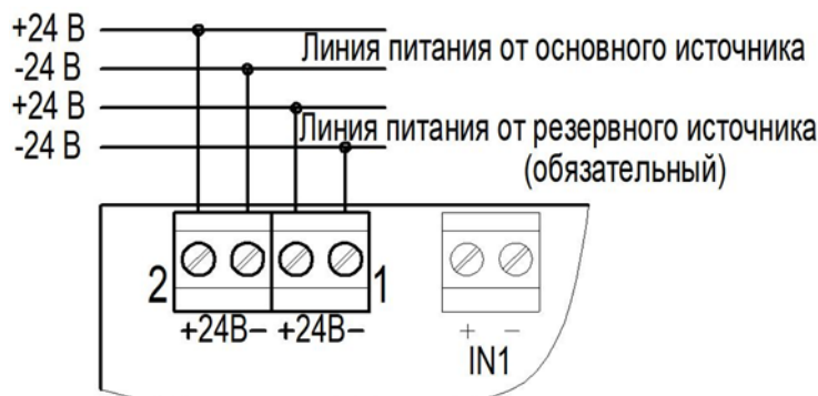
Рисунок 10 – Подключение питания
