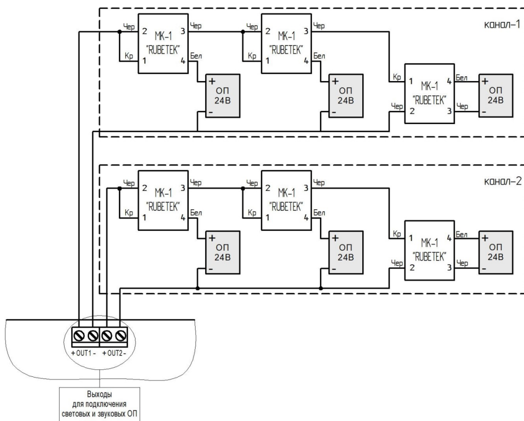
Рисунок 12 – Схема подключения СОУЭ
