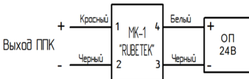
Рисунок 13 – Схема подключения МК-1 к ОП
