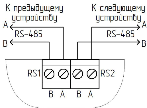
Рисунок 9 – Подключение RS-485
