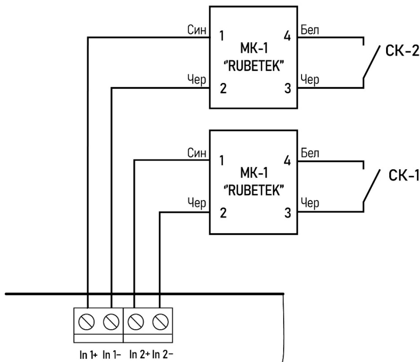
Рисунок 15 – Схема подключения свободно программируемых входов
