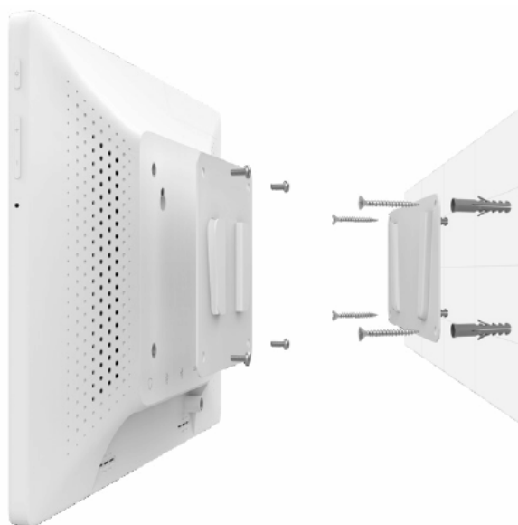
Рисунок 5 - Монтаж панели
