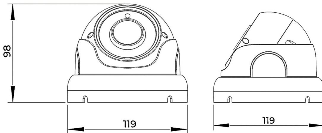
Рис. 2 – Габаритные размеры видеокамеры
