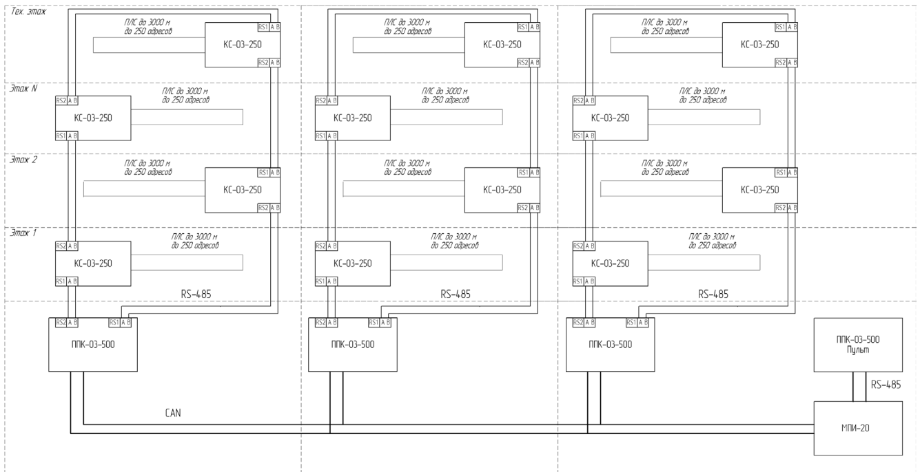
Рисунок 4 - Схема организации интерфейса RS-485
