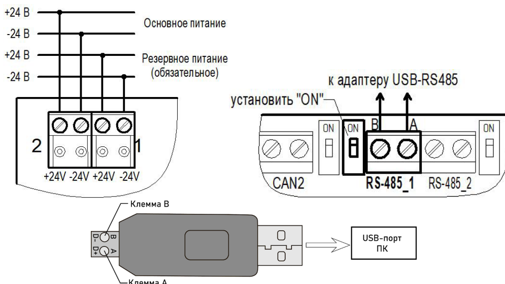
Рисунок 8 - Схема подключения адаптера USB-RS485
