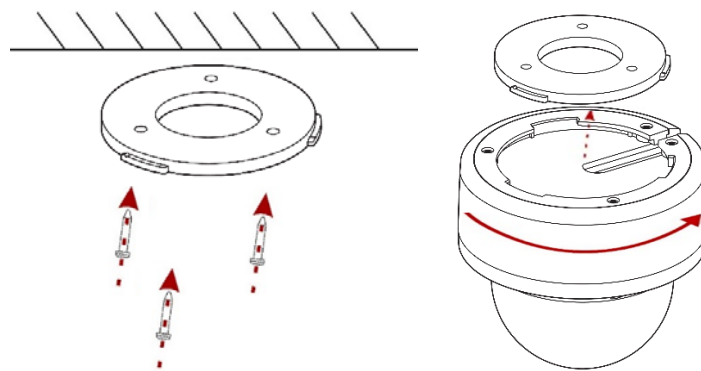
Рис. 1 – Монтаж камеры
